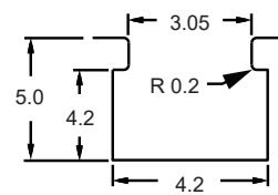
GROOVE DIMENSIONS
