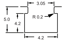
GROOVE DIMENSIONS
