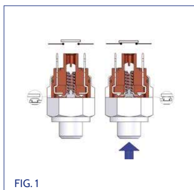
(esempio di funzionamento non vincolante - contatto N.A.) (non-binding example - N.O. contact)
